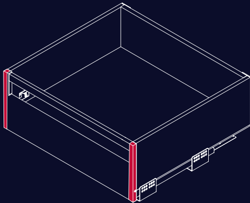
Крепление передней панели EVA Slimbox H=167 (C)/H=199 (D)
