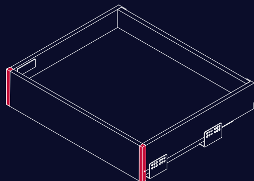
Крепление передней панели EVA Slimbox Н=84 (М)
