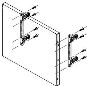
Установка держателей фасада
