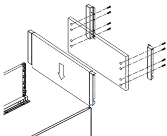
Установка держателей фасада
