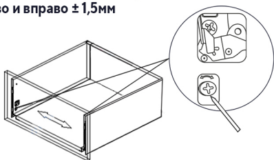
Регулировка фасада по вертикали Вверх и вниз \pm 1,5 мм
