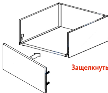
Установка фасада
