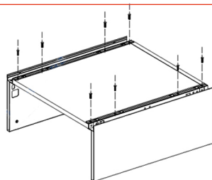
Установка дна ящика
